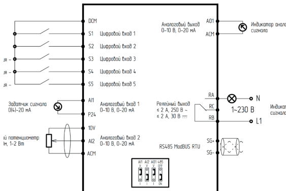
Рисунок 4 – Подключение управляющих клемм для преобразователя частоты серии LCI(S)
