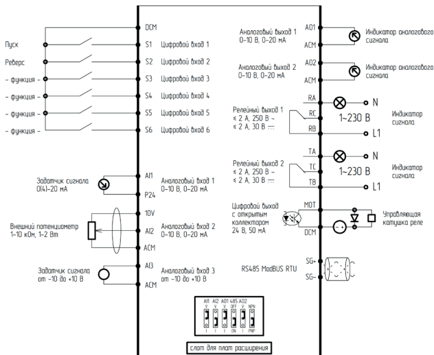
Рисунок 5 – Подключение управляющих клемм для преобразователя частоты серии LCI
