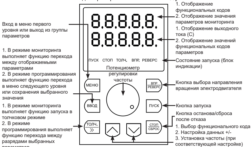
Рисунок 7 – Описание панели управления LCI-KP
