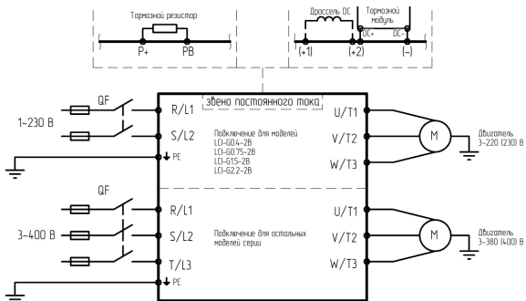
Рисунок 3 – Подключение силовых клемм для преобразователя частоты серии LCI
